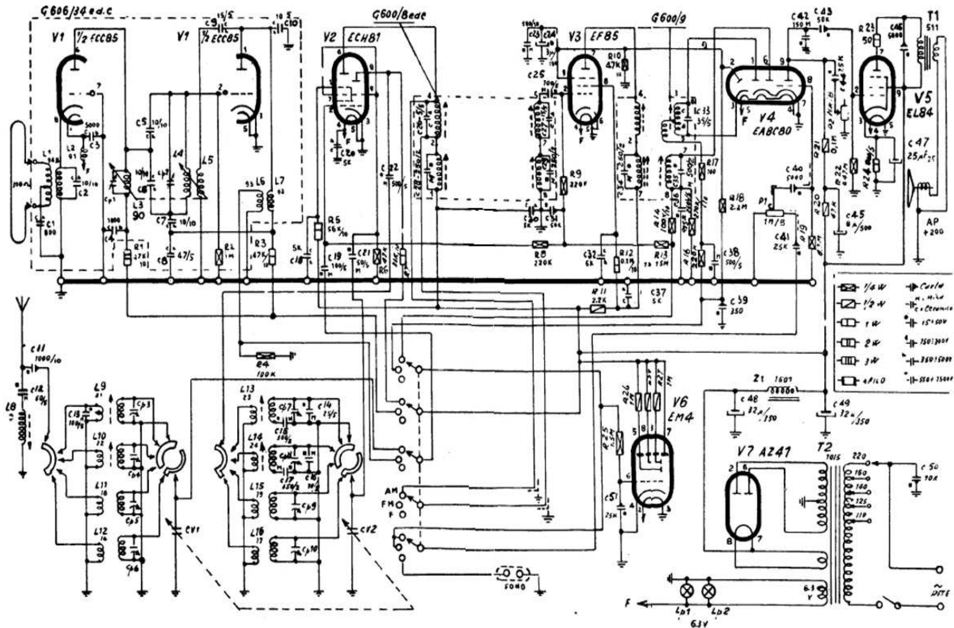
ALLOCCIO BACCHINI - Mod. 316 B. Apparecchio a modulazione di ampiezza e di frequenza, con cinque gamme di ricezione, una OM, tre OC e una UC a FM. Media frequenza AM a 465 kc/s, e FM a 10,7 Mc/s. Potenza d'uscita 4,5 watt e potenza assorbita 60 VA.
